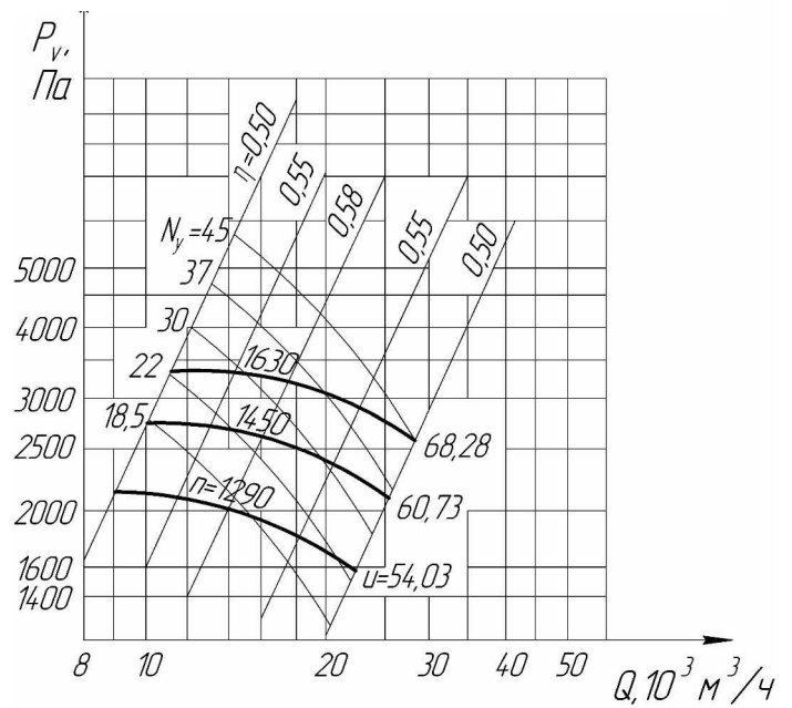
ВРП115-45-8
